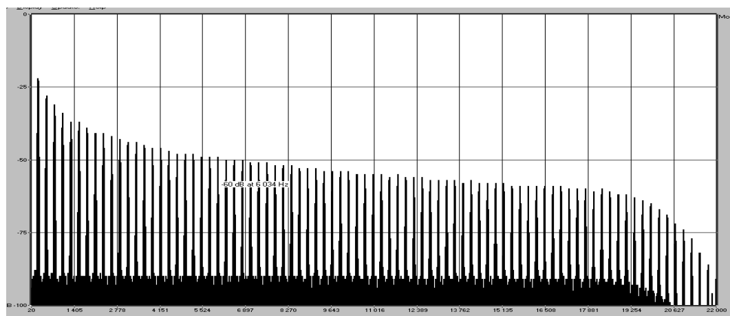
Spectre de réponse fréquentielle du Modular V intégrant la technologie TAE
