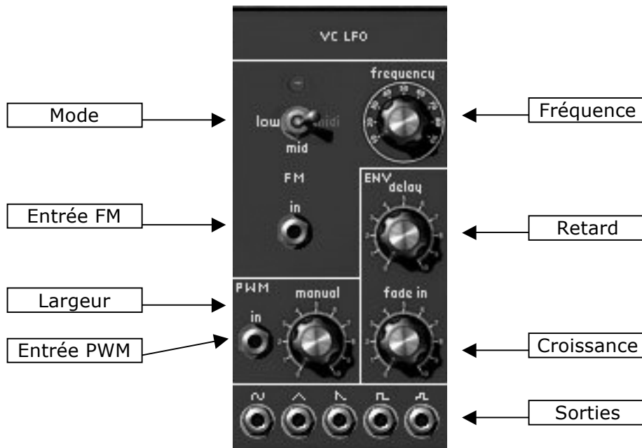
Oscillateur basse-fréquence
