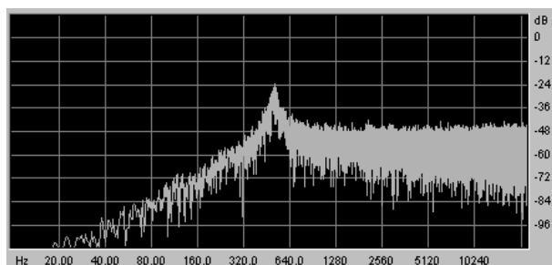
Passe-haut 12 dB/octave
