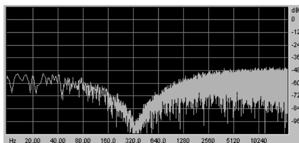
Coupe-bande 24 dB/octave
