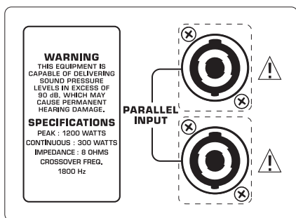
Afb. 1.1: Aansluitingen op de B1520 PRO (vergelijkbaar met B2520 PRO/B1220 PRO)
