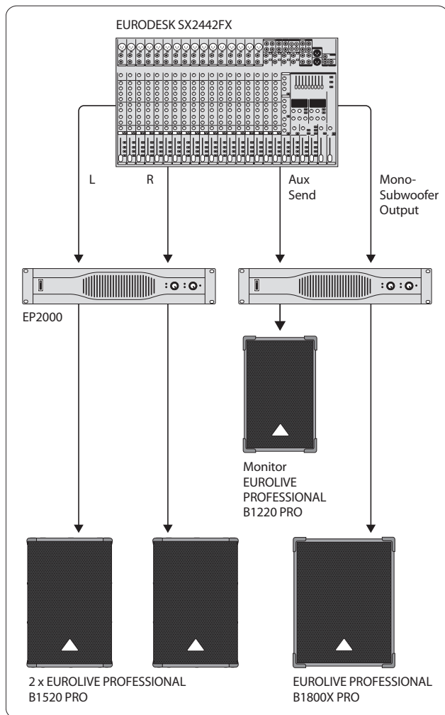
Afb. 6.1: Stereoweergave met parallelle podiummonitor en subwoofer
