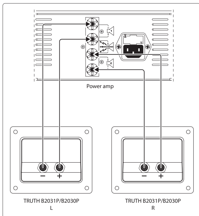
Fig. 3.1: Collegamento ad un amplificatore
