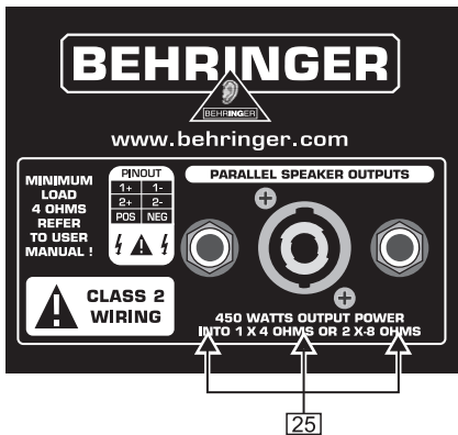
Рис. 2.5: Обратная сторона BX4410/BX4410A (отрезок 2)
