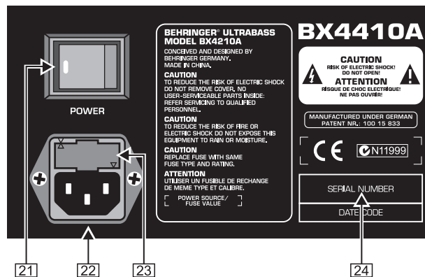
Рис. 2.4: Обратная сторона BX4410/BX4410A (отрезок 1)
