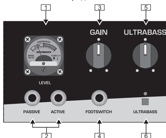
Рис. 2.1: Передняя часть BX4410/BX4410A (сектор 1)
