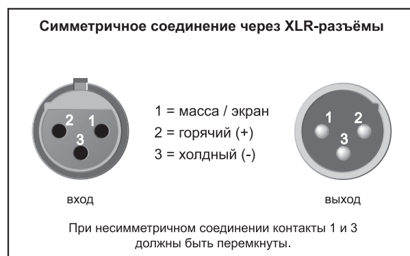
Рис. 73: XLR-соединения
