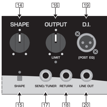
Рис. 2.3: Передняя часть BX4410/BX4410A (сектор 3)
