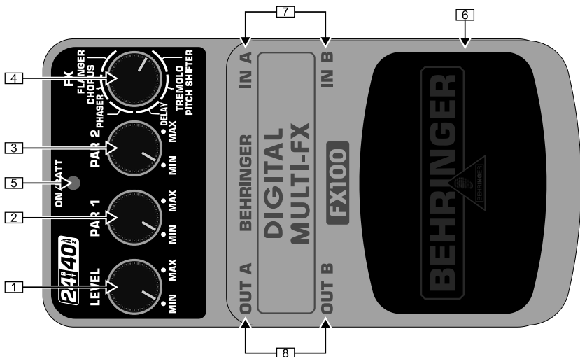
Aanzicht bovenkant
