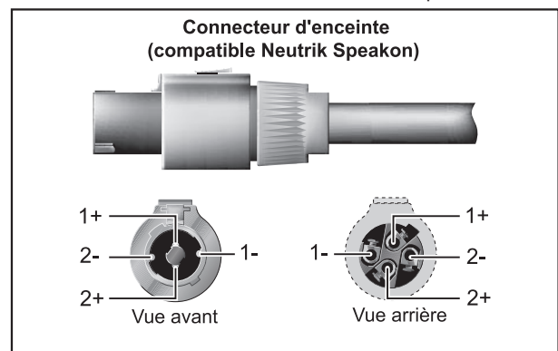
Fig. 2.3: Connecteur professionnel compatible Neutrik Speakon
