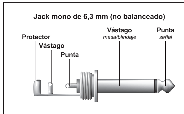
Fig. 2.2: Conector de altavoz tipo jack mono de 6,3 mm
