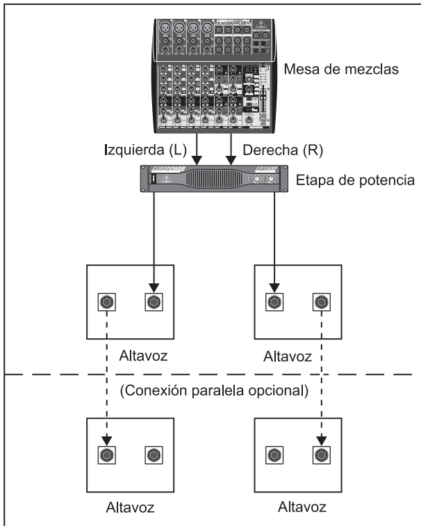
Fig. 4.1: Operación estéreo con altavoces de rango completo
