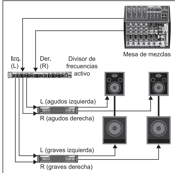
Fig. 4.2: Operación estéreo a 2 vías con subwoofers
