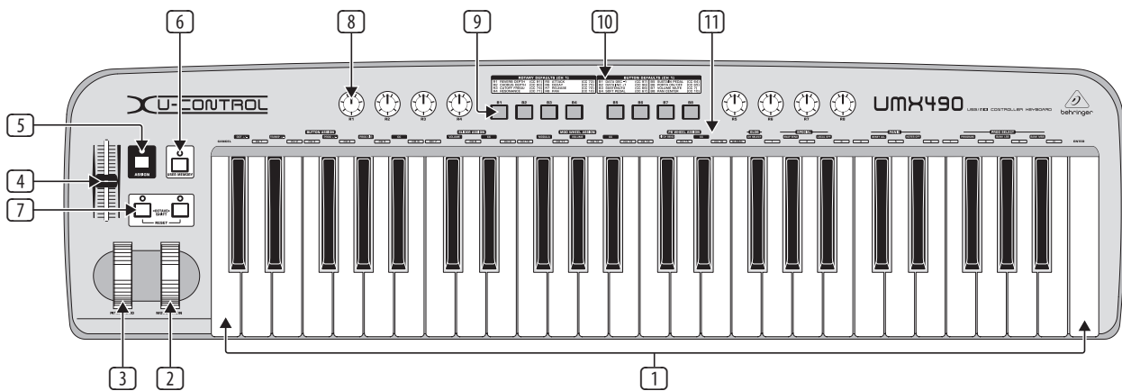
图 3.1 俯视图
