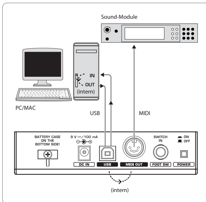
图 2.1 MIDI 信号流向图
