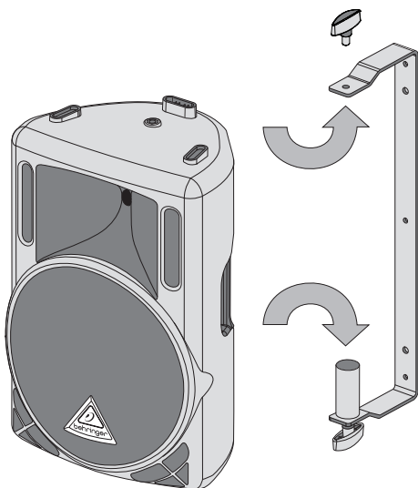
Fig. 1 : Fixez le baffle dans l'arceau de montage
