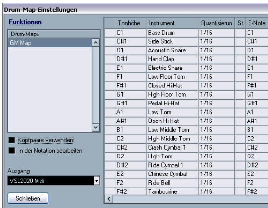
Der Dialog »Drum-Map-Einstellungen«
